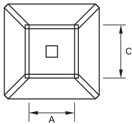
沓石
