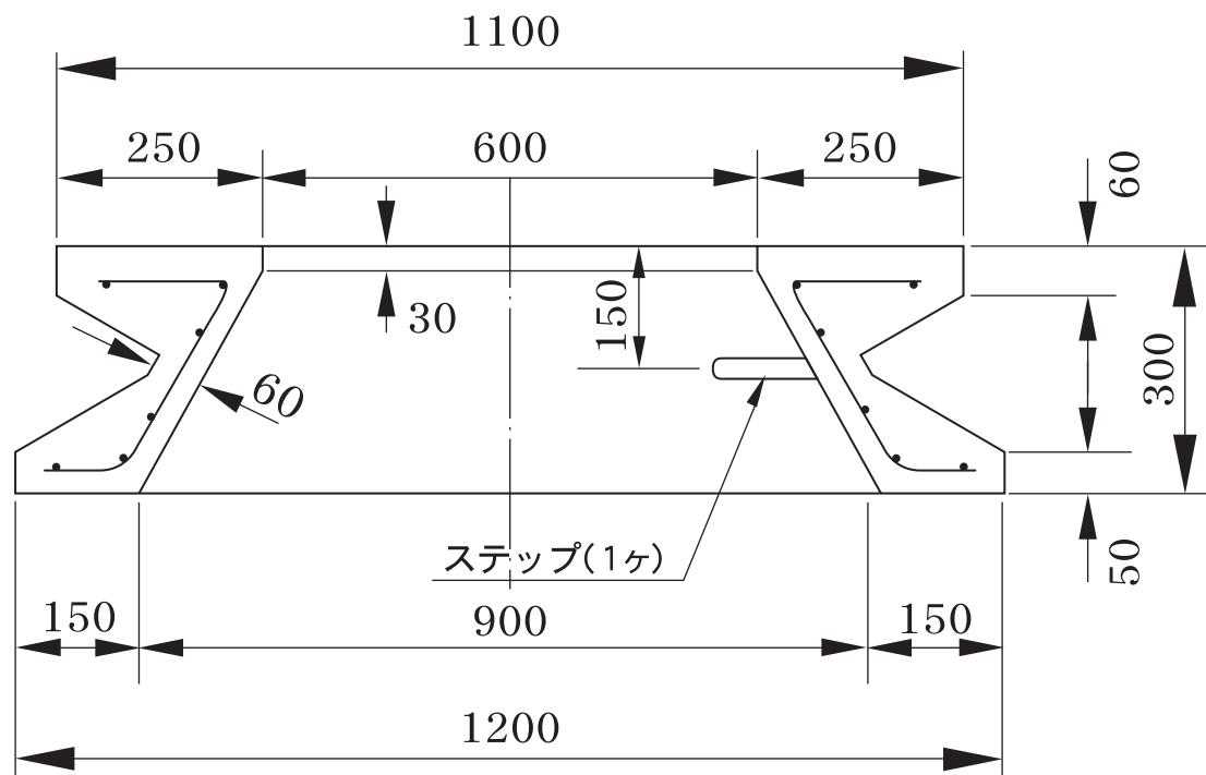
A-A 断面図
