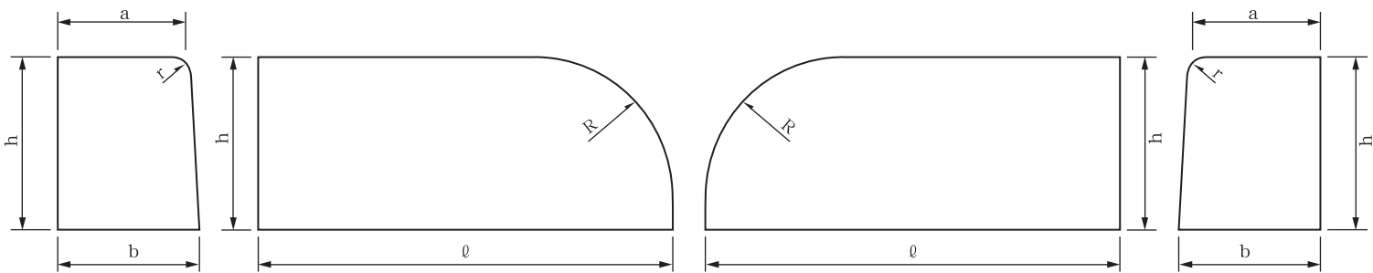
● 歩車道境界端末ブロックB 右
