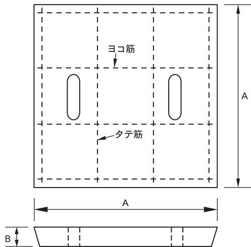
仕様寸法表 (単位 mm)
