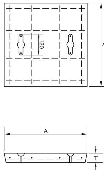
汚水蓋
