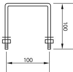
汚水手掛け金具 9φ
