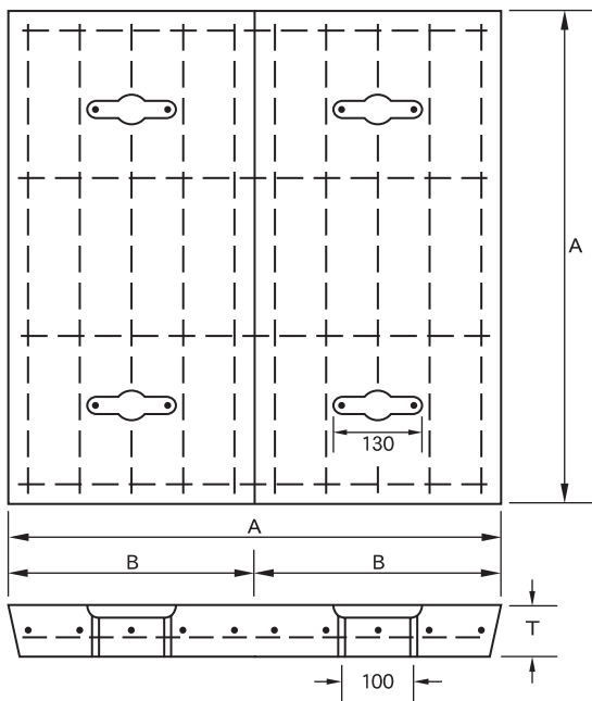
汚水蓋 600
