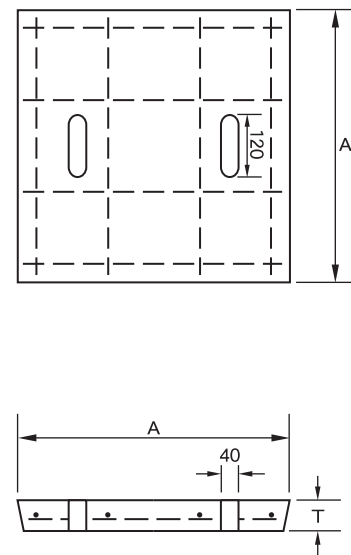
雨水蓋
