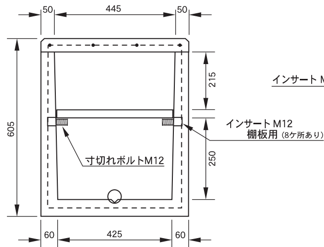
・横断面図
