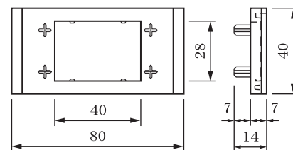
● 反射板付プレート詳細図
