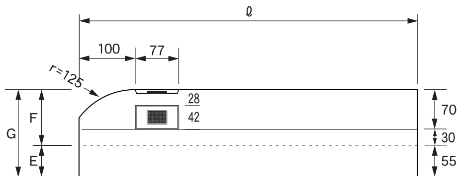
● 正面図 (右)
