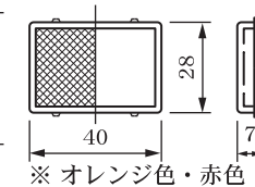
● 反射板詳細図
