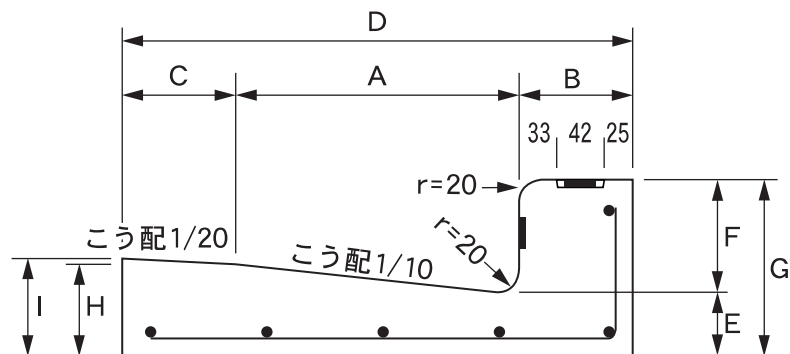
● 側面図 (左)
