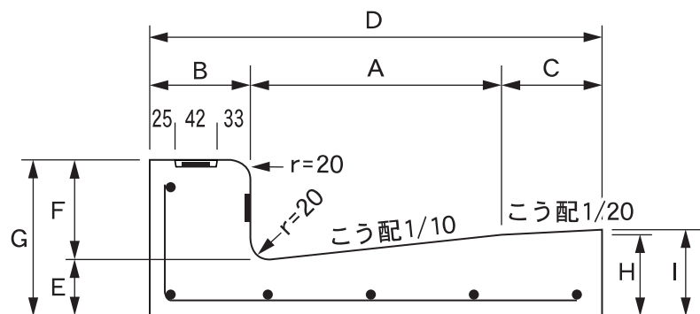
● 側面図 (右)
