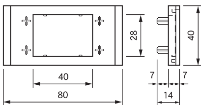
反射板取付プレート詳細図
