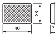
反射板詳細図
