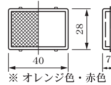
● 反射板詳細図
