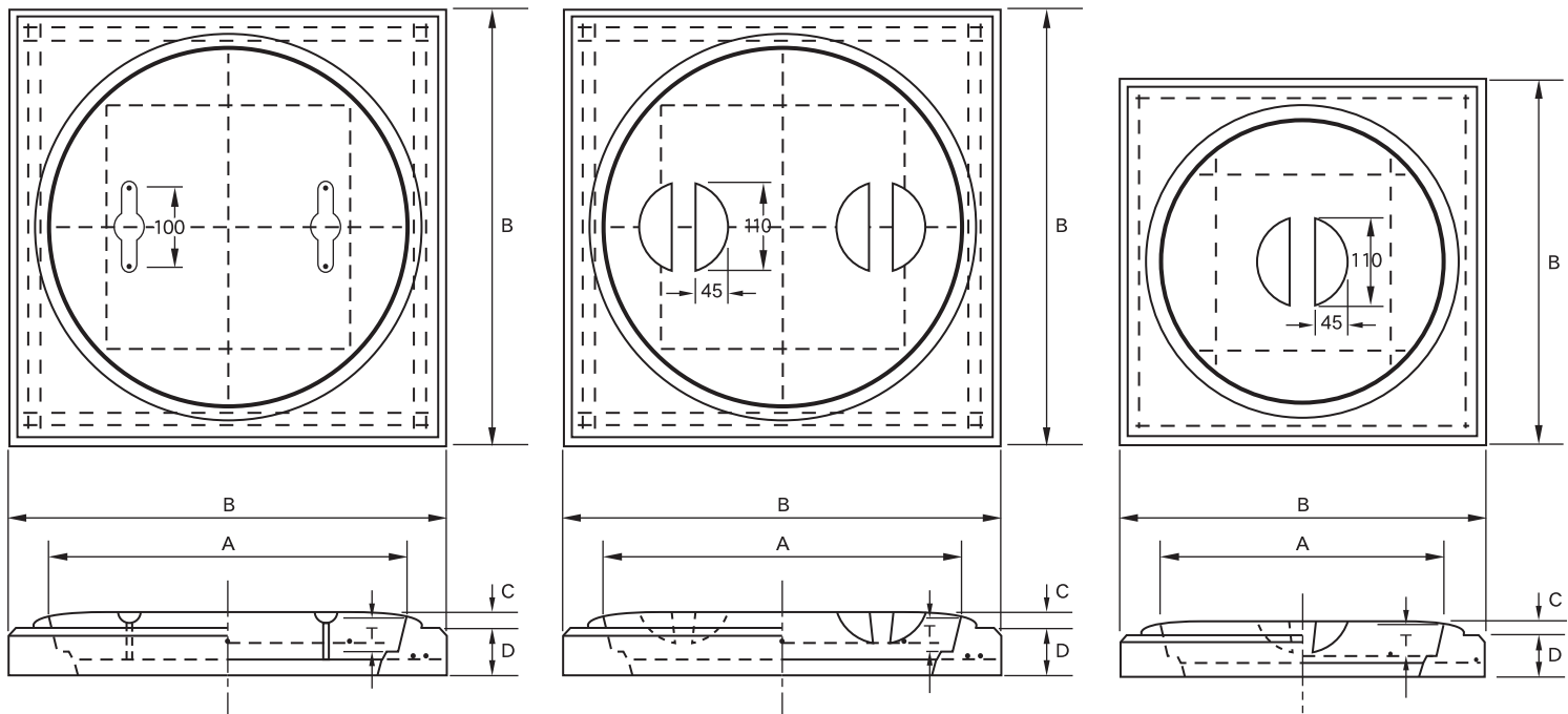
600用マンホール蓋
