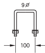
マンホール蓋手掛金具
